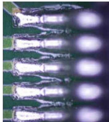
b) SAC0307
