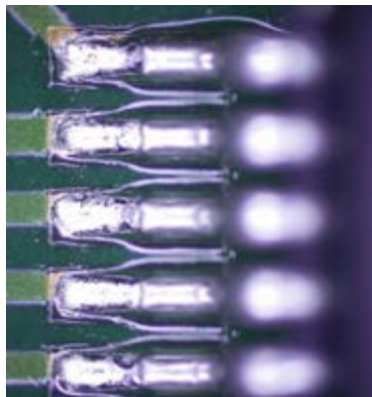
a) SAC305
