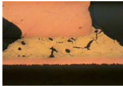
SAC0307
