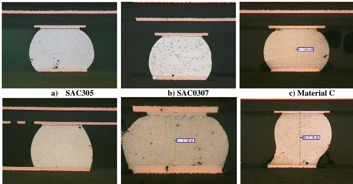
d) SnCuNi e) Material D f) SnBiAg
